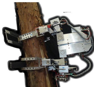
木登りロボット Woody-2
